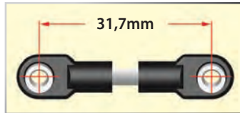
Vorlage: Lenkungsverbindungs-länge
