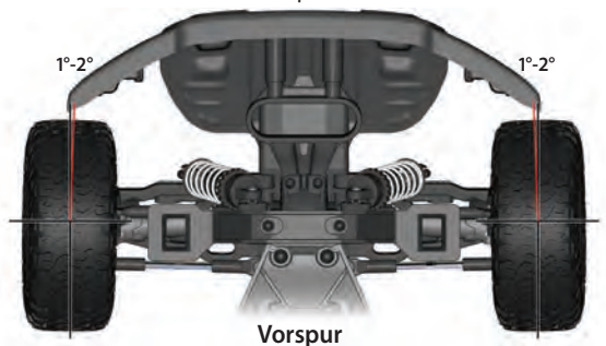
Vorspur
