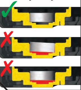
Linke Getriebehälfte
